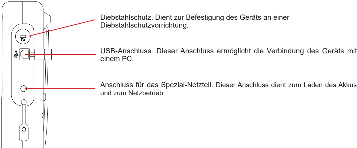
Abbildung 5: Seitliche Anschlüsse
