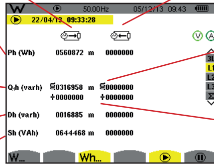
Abbildung 102: Bildschirm zur Anzeige der verbrauchten und erzeugten Energien bei L1
