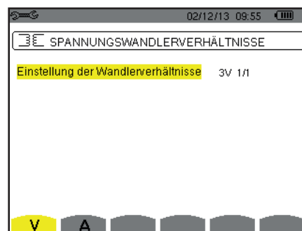
Abbildung 28: Bildschirm Spannungsverhältnisse im Menü Stromwandler und Übersetzungsverhältnisse – Fall einer Anordnung mit Neutraleiter
