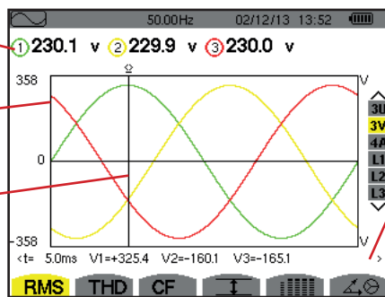
Abbildung 54: Bildschirm zur RMS-Anzeige bei 3V
