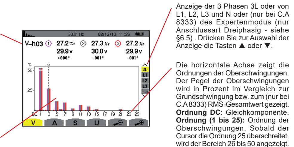
Abbildung 42: Anzeigebeispiel für Oberschwingungen der Phasenspannung bei 3L
