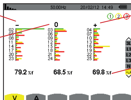
Abbildung 50: Bildschirm des Expertenmodus für die Phasenspannung (dreiphasige Anordnungen mit Neutralleiter)
