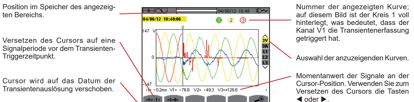
Abbildung 40: Beispiel für die Anzeige von Transienten in Form von Kurven bei der Anschlussart Dreiphasig 4 Leiter
