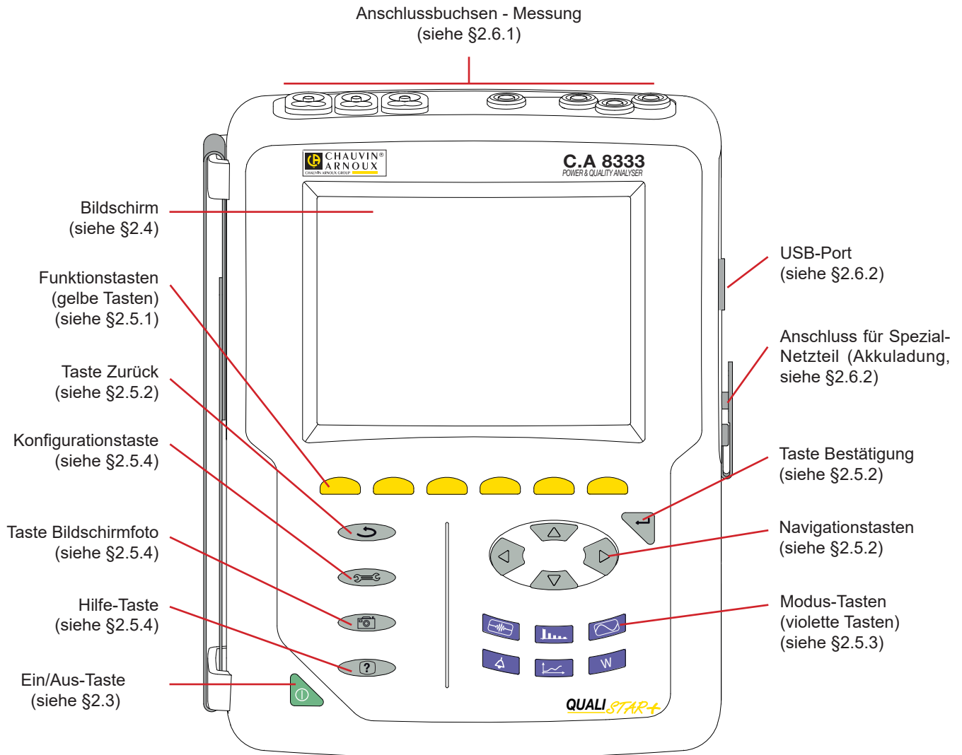
Abbildung 2: Gesamtansicht des Qualistar+
