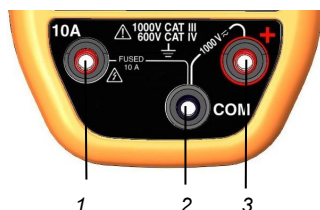
Figure 4 : les bornes
