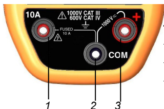
Abbildung 4 : die Buchsen
