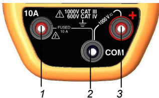
Figura 4: i morsetti
