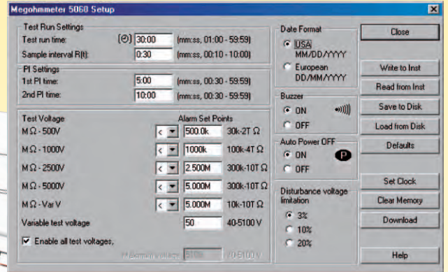
Configuración simple y fácil a través de una sola ventana de diálogo.
