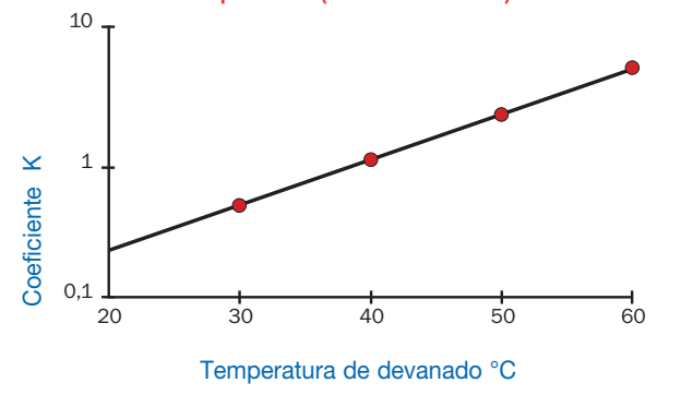
Corrección de la resistencia del aislamiento en función de la temperatura (fuente IEEE - 43)
