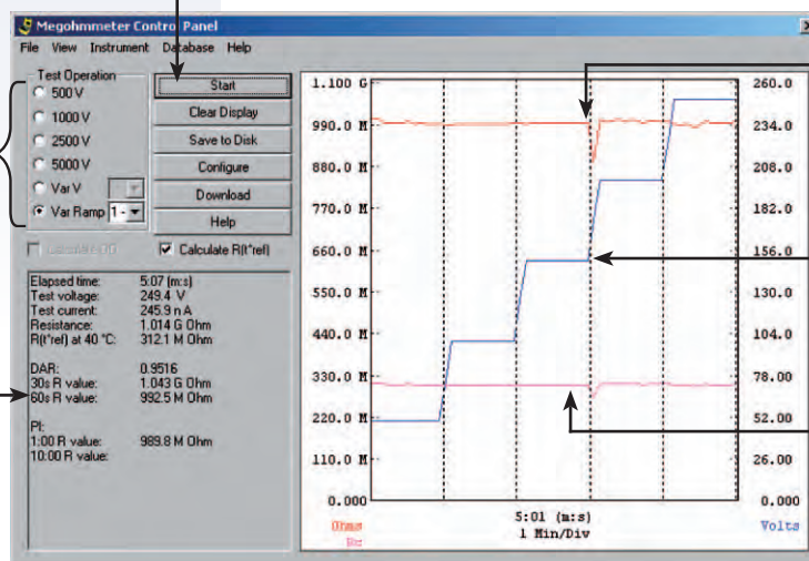
Inicio del test y resultados (texto y gráficas) agrupados en un mismo cuadro de diálogo en el modelo C.A 6549. También se muestran los saltos de tensión.
