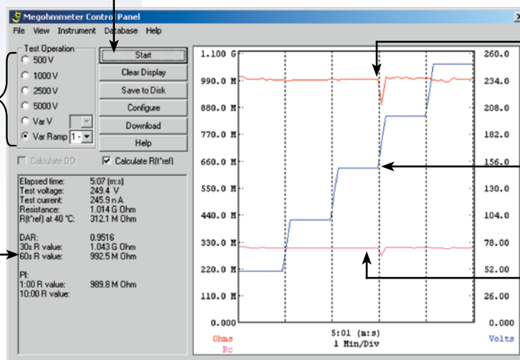
Lancement du test et résultats (textes et graphiques) regroupés dans une boîte de dialogue, pour le modèle C.A 6549, les pas de tension sont également affichés.
