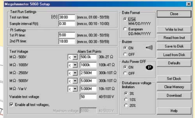
Configuration simple et facile par une seule boîte de dialogue.
