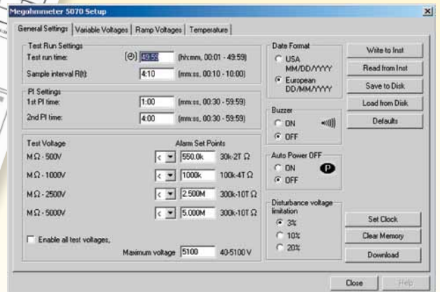
La boîte de dialogue à quatre onglets permet une configuration claire et simple de l'ensemble des fonctions du C.A 6549, y compris pour la programmation des tensions d'essai, des valeurs d'alarme, des pas de tensions et de la compensation de température.
