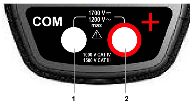
Figura 5 : Los bornes
