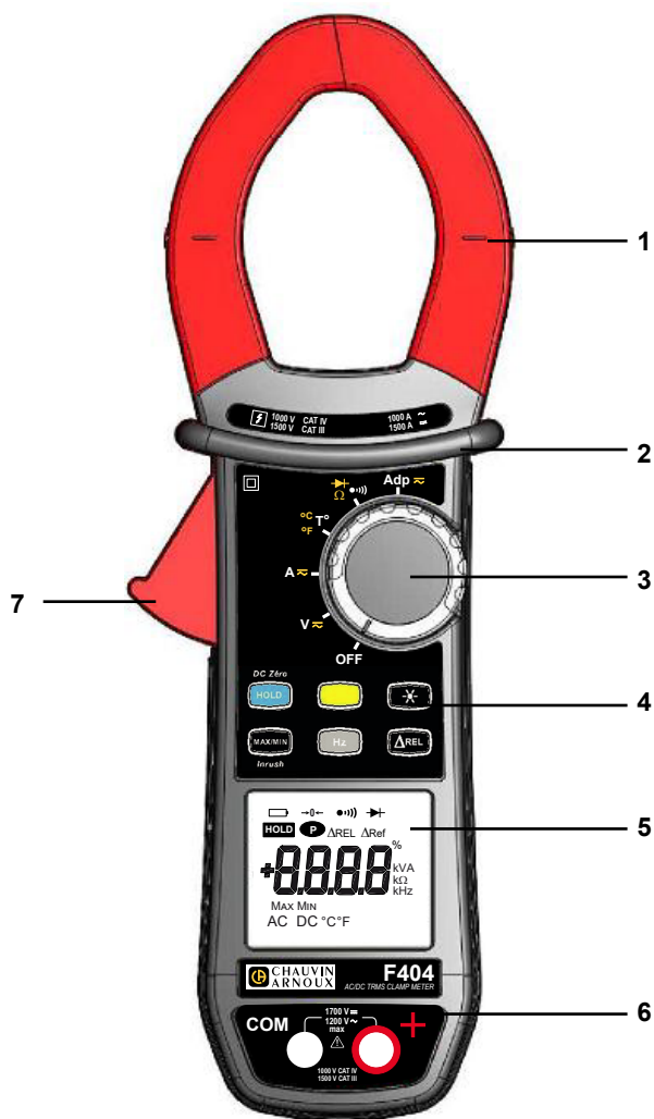
Figura 1 : la pinza multimétrica F404
